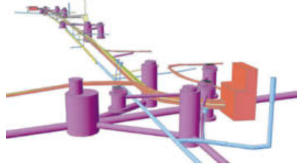
BIM-Modell Werkleitungen Kusenstrasse Küsnacht
